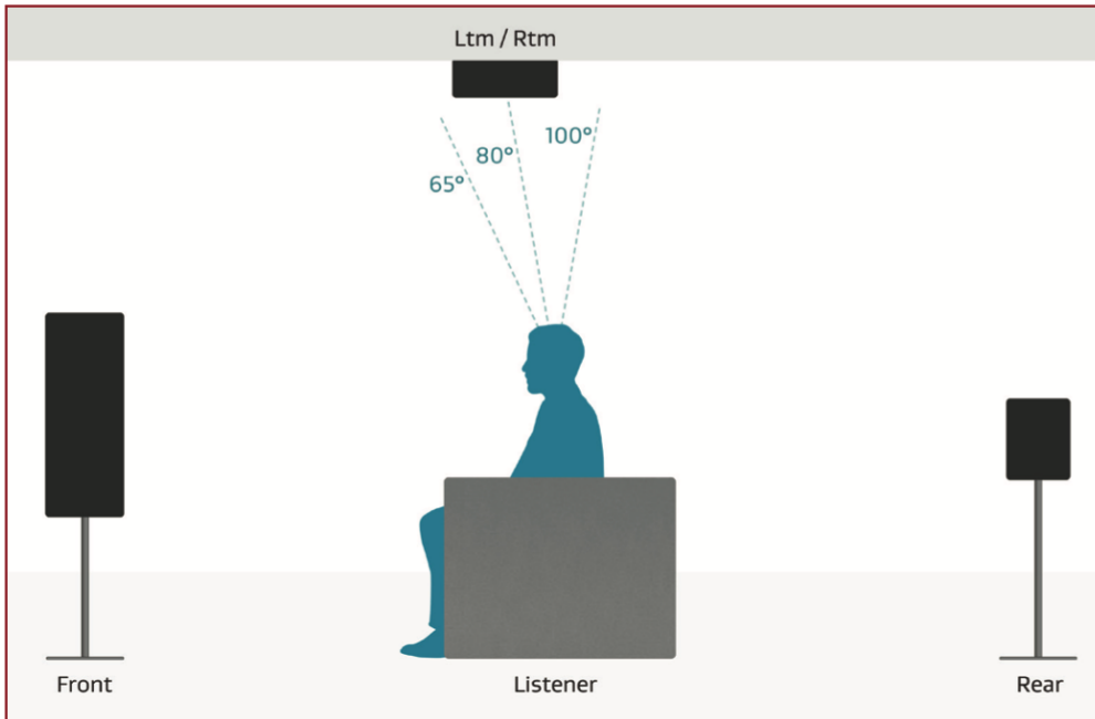
Ein Paar Deckenlautsprecher (Seitenansicht)
